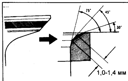
Выпускной клапан.
