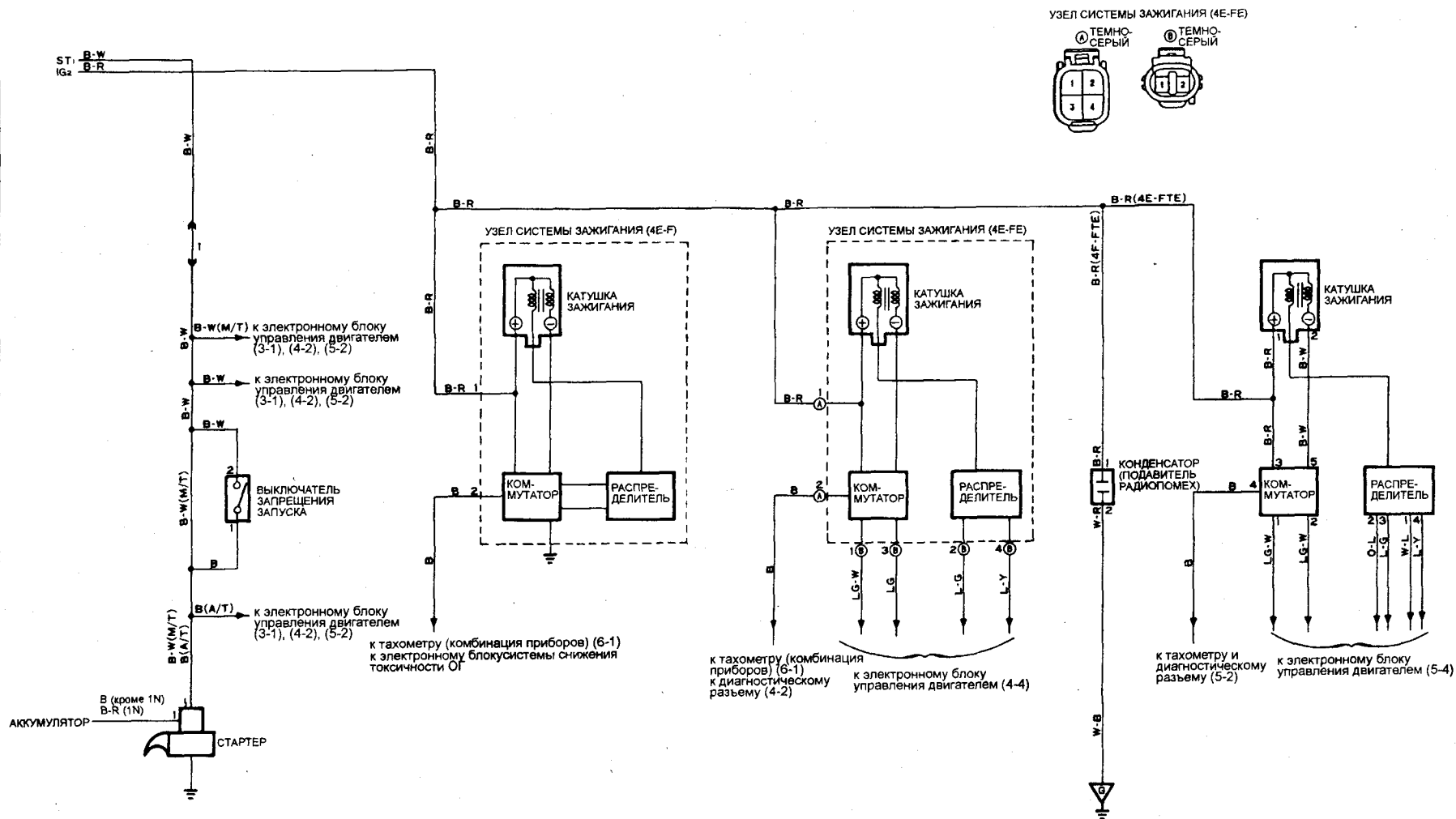
Схема 1-1 (Starlet 80)
