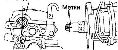
Распределительный вал
