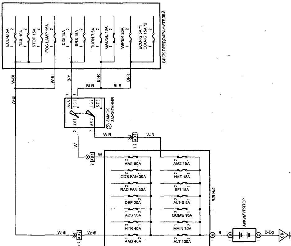
Схема 3-1 (Raum).
