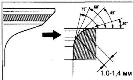
Впускной клапан.
