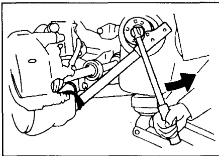
б) Снимите шкив коленчатого вала.
