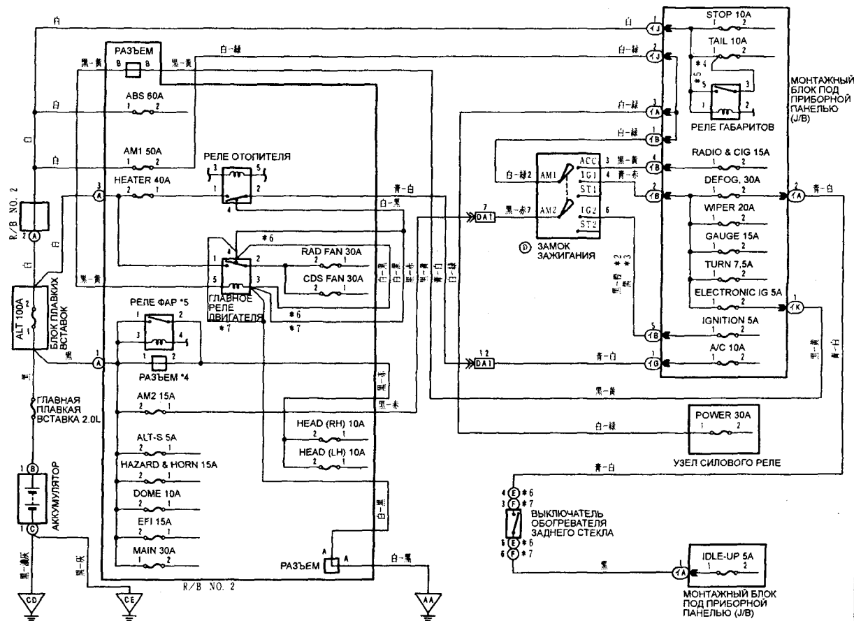
Схема 2-6 (Tercel 50).
