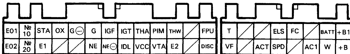
5E-FE (Corolla 100 внутреннего рынка, МКПП).
