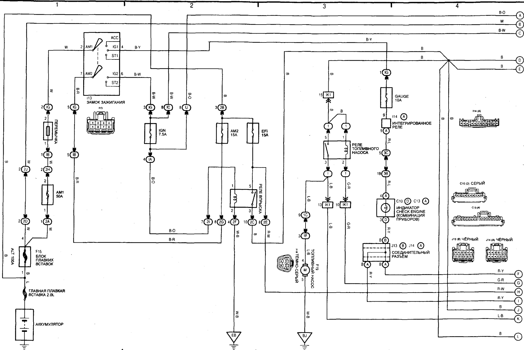
Схема 5-2 (Corolla 110, модели внешнего рынка).
