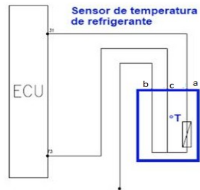
Figura 2: Diagrama del sensor ECT; Fuente: ref. (4)
